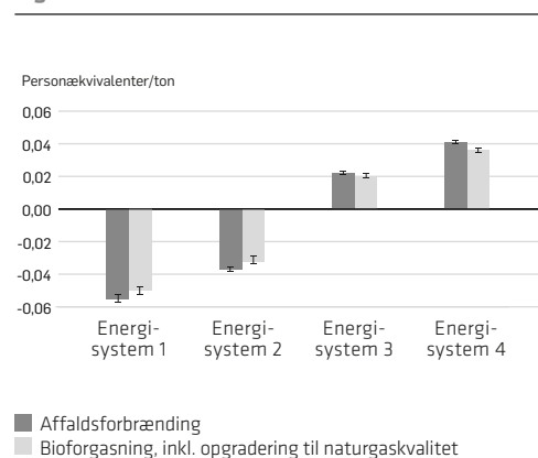
Figur 7.3.3 Netto drivhuseffekt
