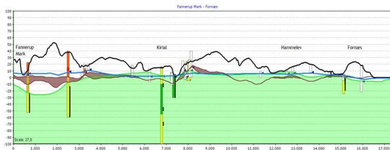
Figur 3.4 - Geologisk tværsnit fra Fannerup til Fornæs.
